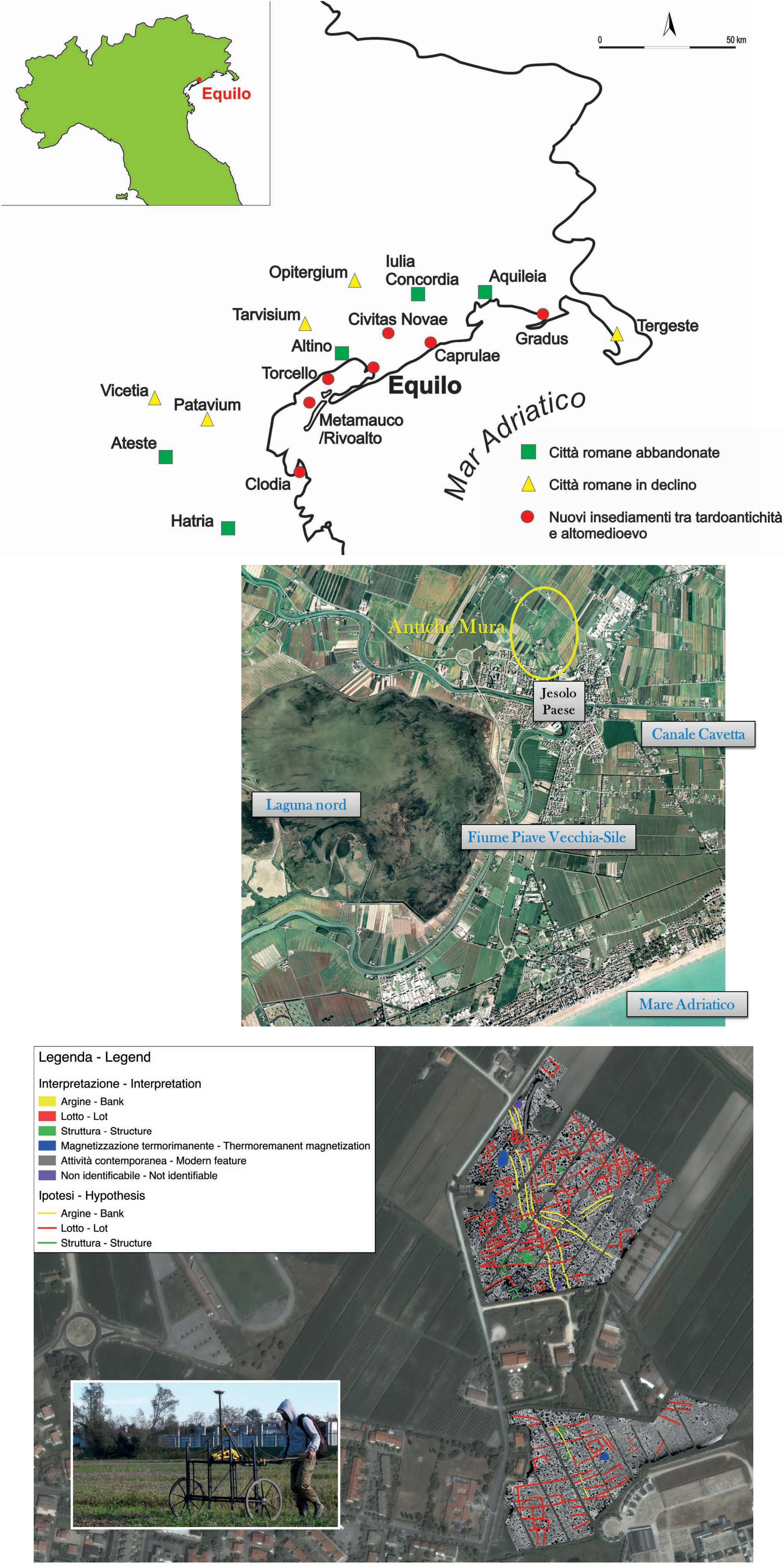
L’interpretazione delle tracce registrate dal rilievo gradiometrico (il segnale magnetico restituito da strutture e canali presenti nel sottosuolo).
